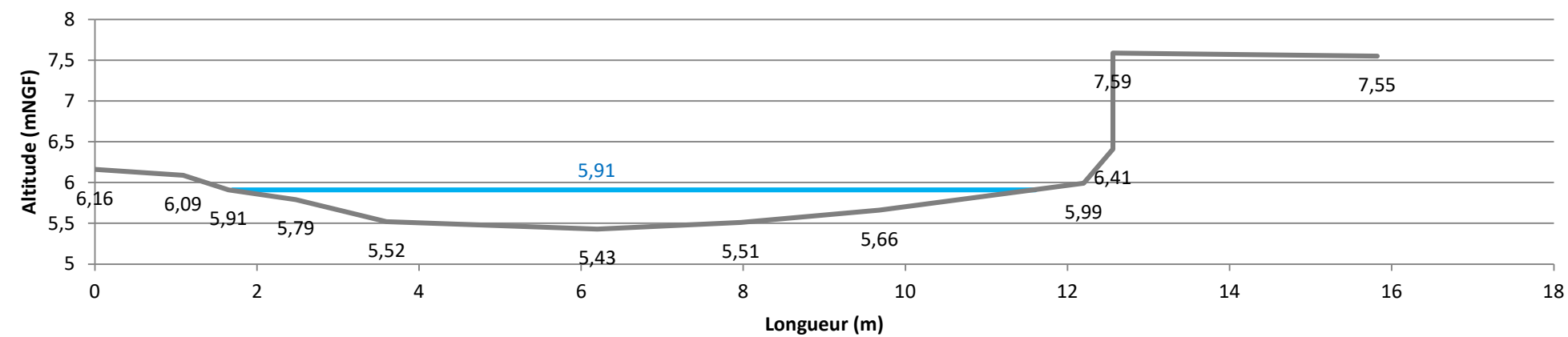
PT 1 - Vannes ouvertes (26/05/2020)
