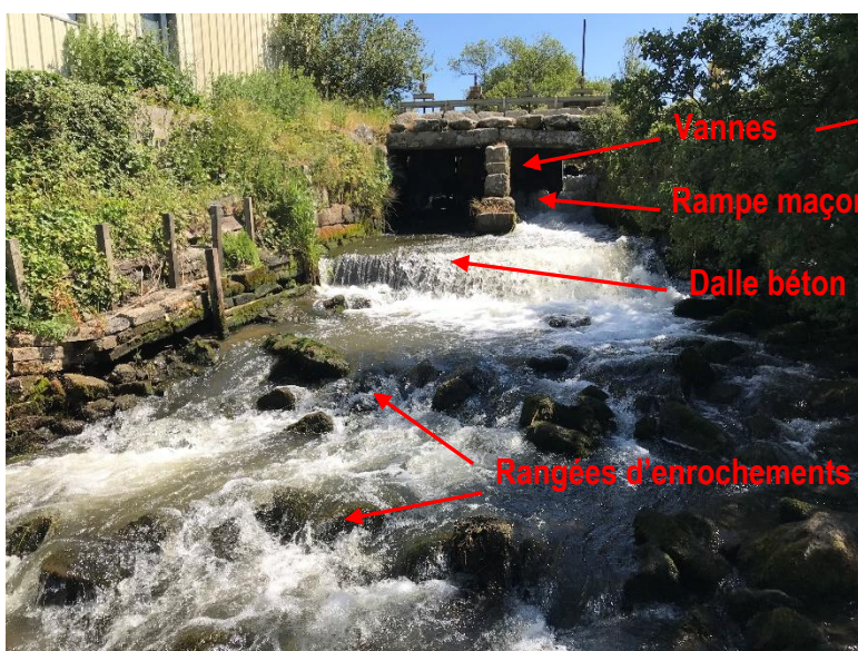
Vue du vannage principal depuis l'aval, montrant la succession d'obstacles simples dont est constitué le radier.
