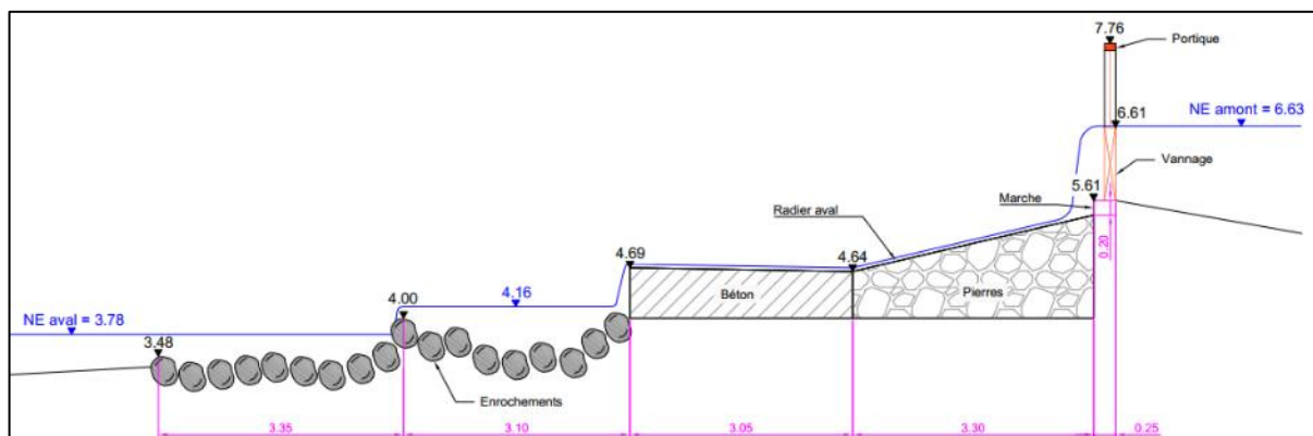
Coupe en long de l'ouvrage principal (voir cahier de plans de l'état actuel).
