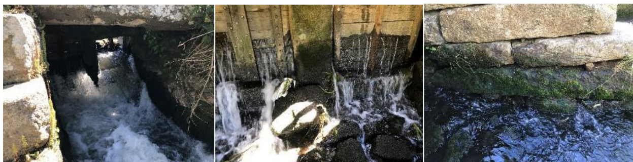
Vannage de gauche détruit - Fuites dans vannes de droite et déchaussement de la rampe du seuil – Fuites au travers du mur de bajoyer central.
