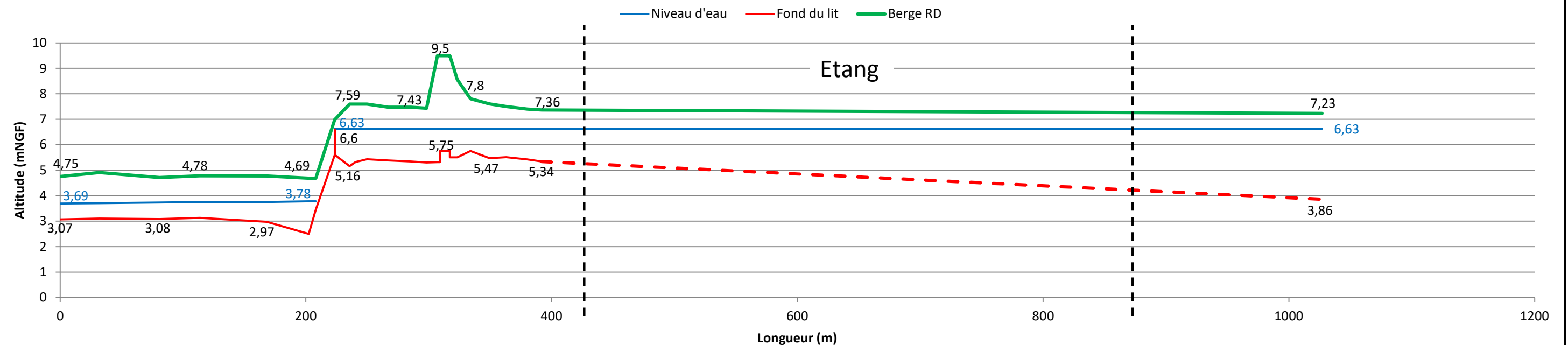
Profil en long - Vannes fermées (22/06/2020)
