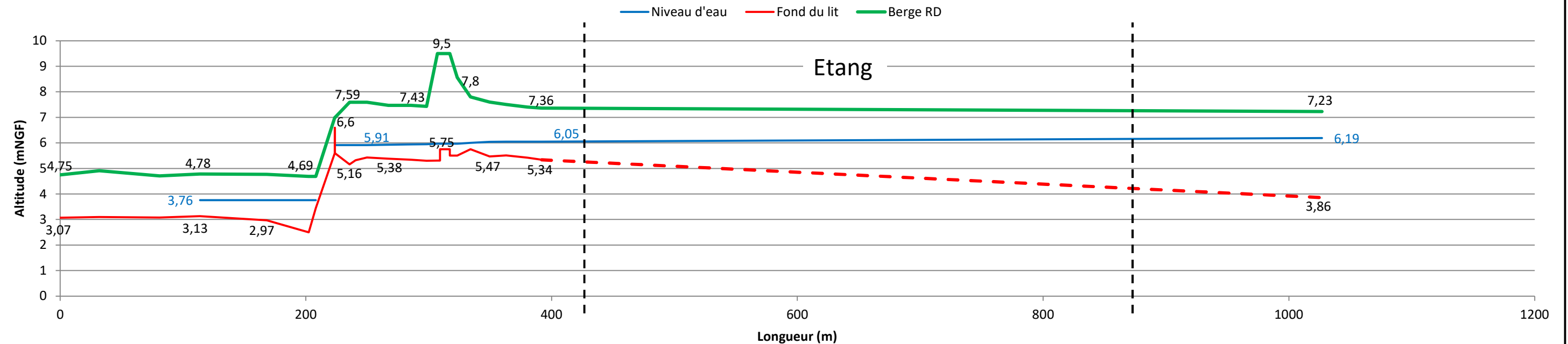
Profil en long - Vannes ouvertes (26/05/2020)
